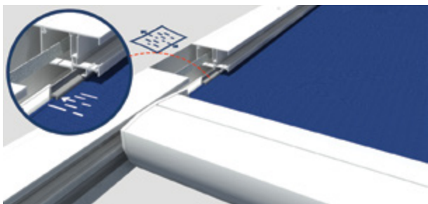
A ZIP screen technológia folyamatos feszítésének köszönhetően a technikai textil szorosan illeszkedik a lefutósínekbe
