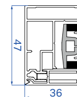
ZIP oldallefutó csavarrögzítéssel
